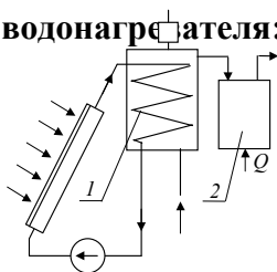
Рис. 2.9 Схема с резервным водонагревателем:
